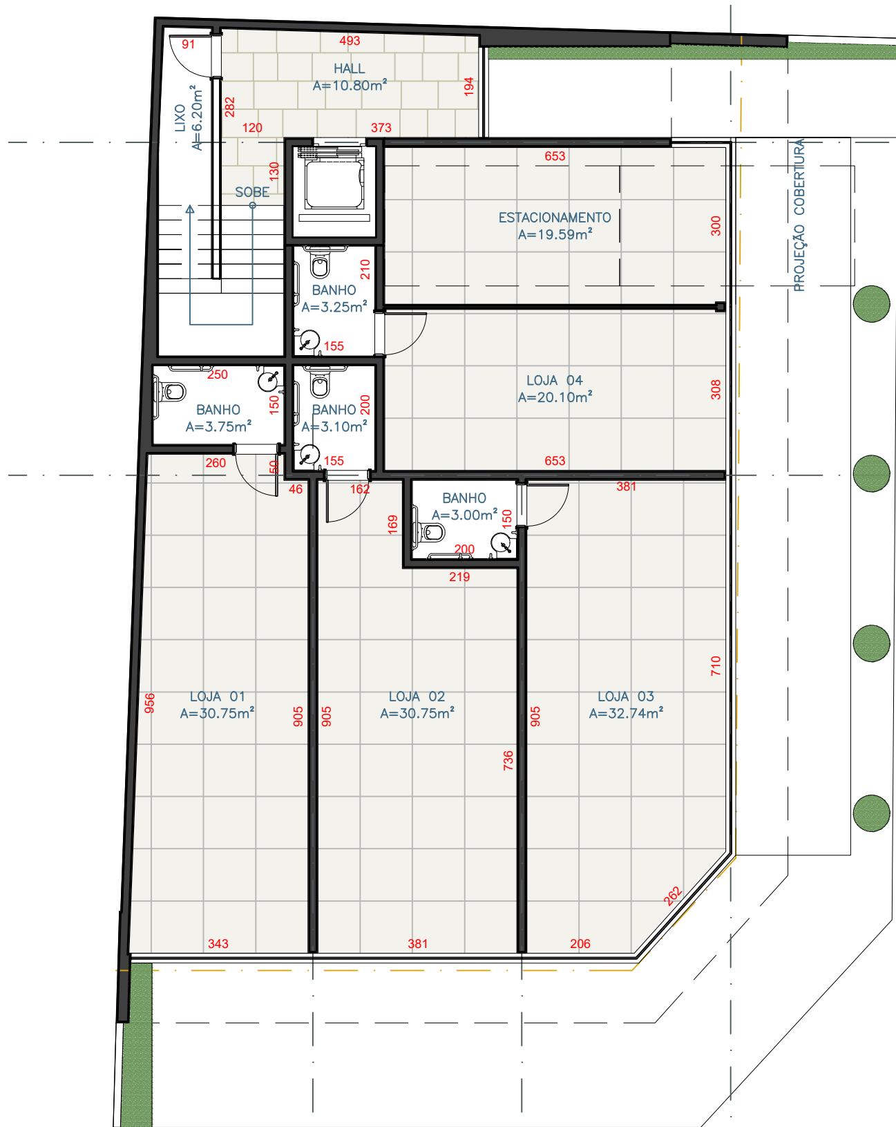
TÉRREO MODELO M1 ESCALA: 1/100
